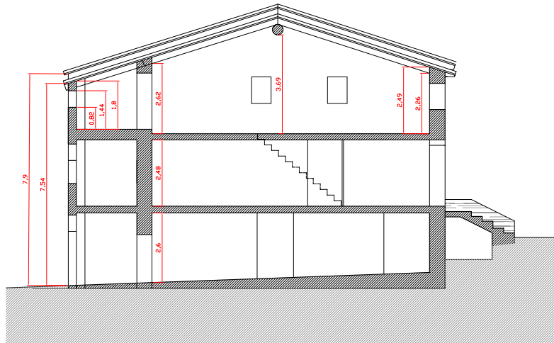
Secció Transversal
