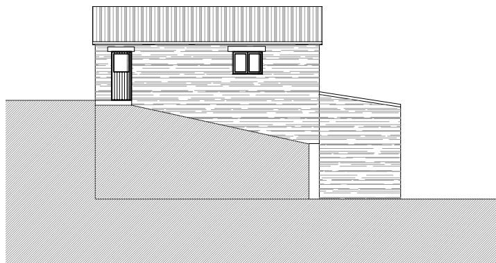
Façana Oest
