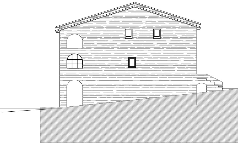
Façana Est
