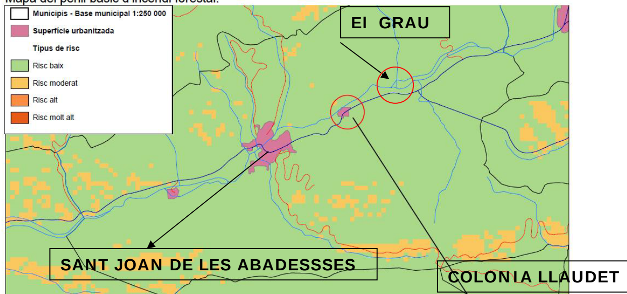
Mapa del perill bàsic d'incendi forestal.
