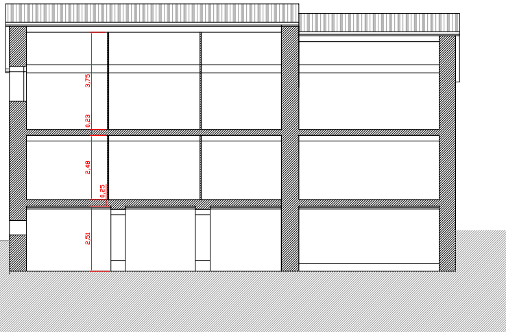
Secció Longitudinal
