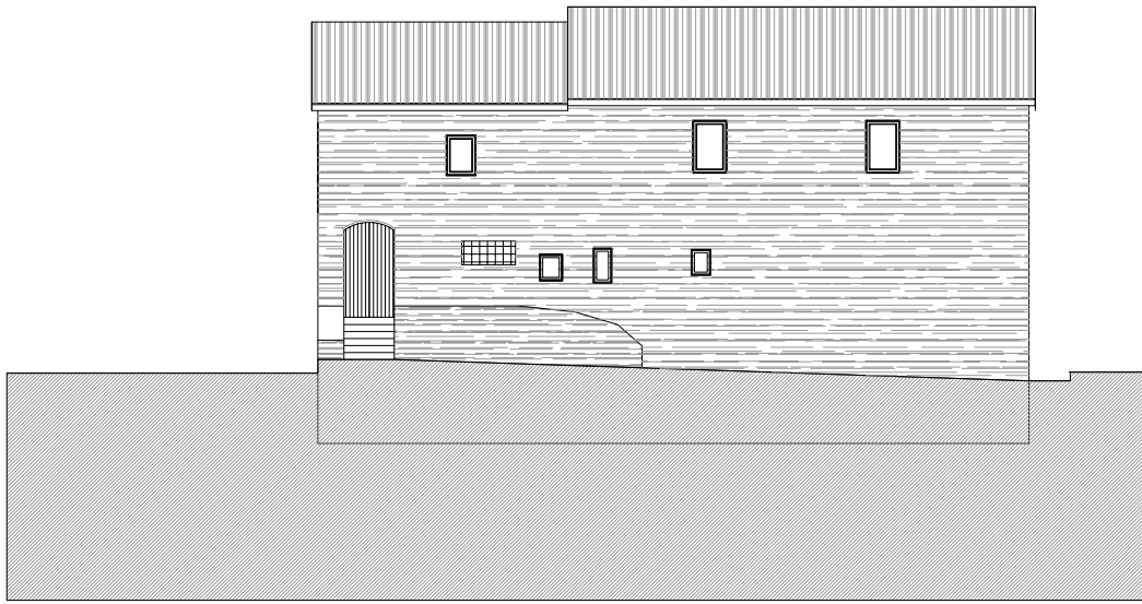
Façana Nord
