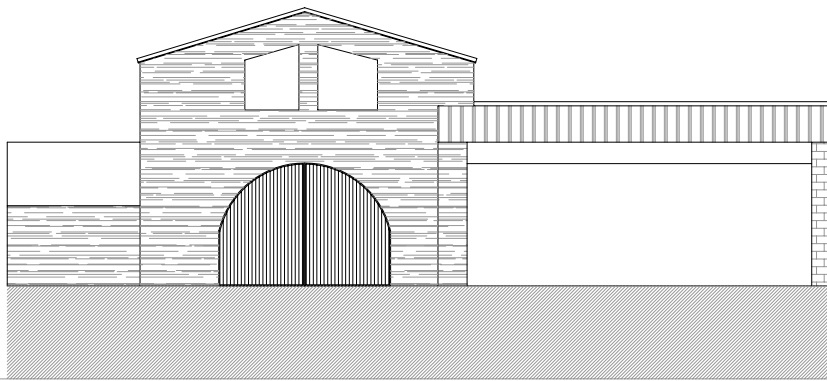
Façana Sud
