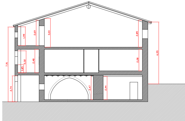
Secció Transversal
