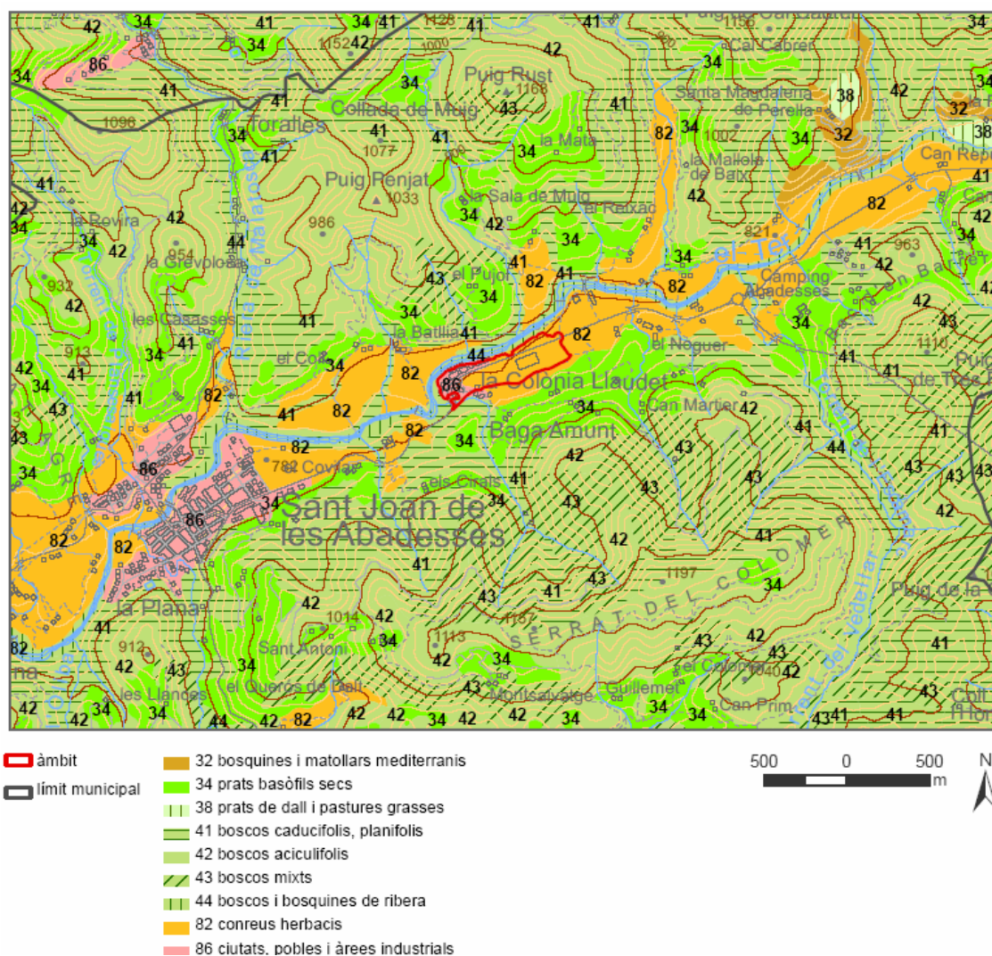
Mapa: Hàbitats presents a l'àmbit i el seu entorn
