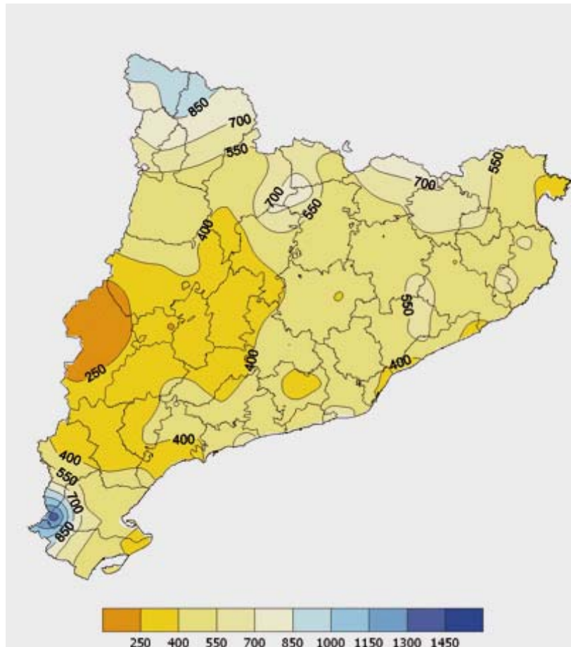
Mapa: Precipitacions anual(mm) Any 2007
