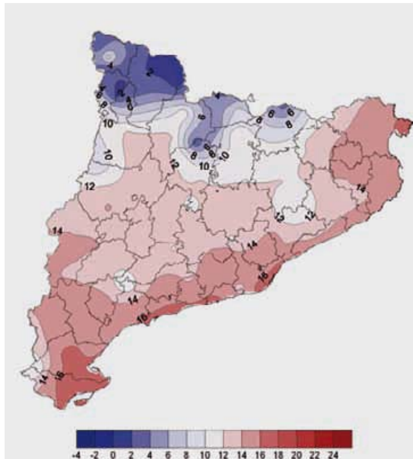
Mapa: Temperatura mitjana anual. Any 2008
