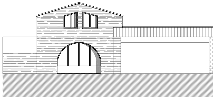
Façana Sud
