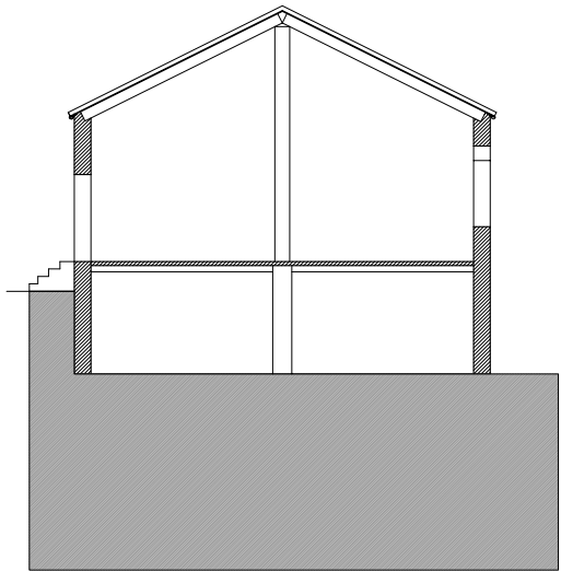
Secció Transversal
